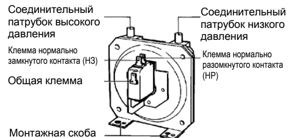
Рис. 6. Общая компоновка реле С6065
