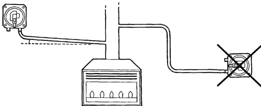
Рис. 7. Слив конденсата
